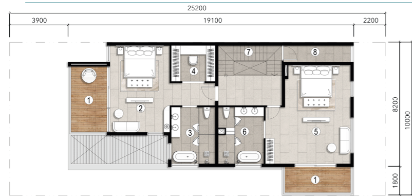
LẦU MỘT / FIRST FLOOR
